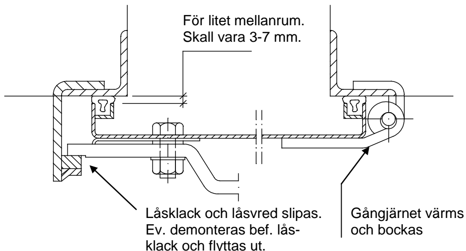
Figur T07-301a. Sektion genom luckblad.
